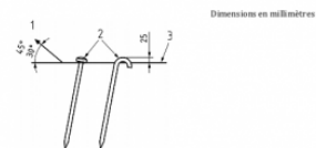
Figure 3 — Exemples de piquets de sol
